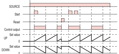
B-2 模式 閃爍 ON start (電源復歸動作)
