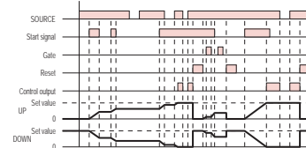
F模式：積算 (電源保持動作)
