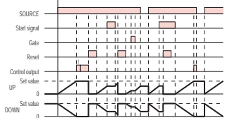
A-2模式：電源 ON 延遲 1 (電源復歸動作)
