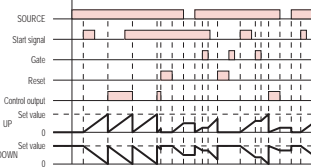
B模式：閃爍 1 (電源復歸動作)
