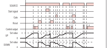
A-3模式：電源 ON 延遲 2 (電源保持動作)
