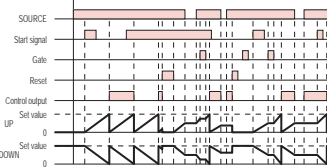
B-1模式：閃爍 2 (電源保持動作)
