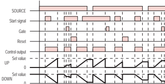
E模式：區間 (電源復歸動作)
