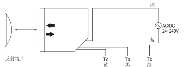
PF系列镜片反射型
